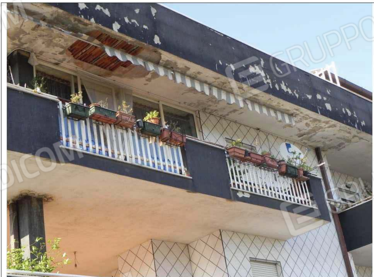
Foto n.4: prospetto lato SUD – particolare pignatte scoppiate
