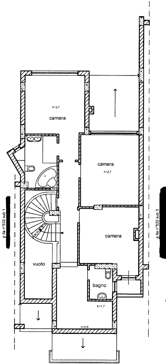
pianta piano primo scala 1:100
