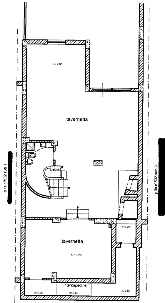
pianta piano seminterrato scala 1:100
