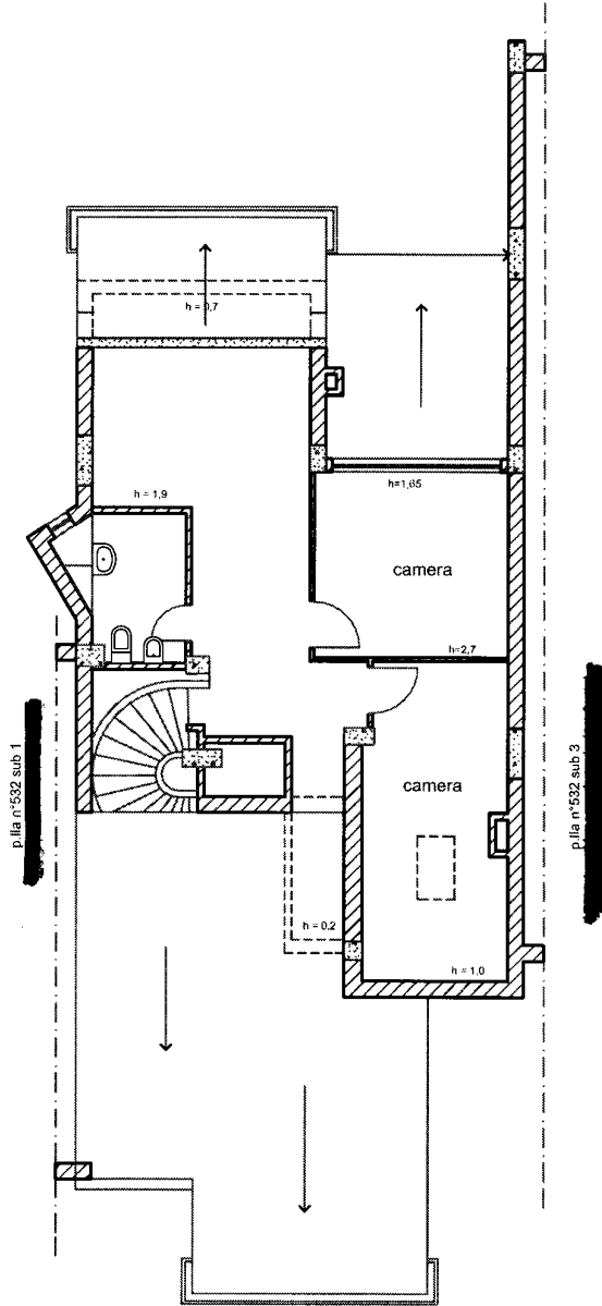
pianta piano sottotetto scala 1:100
