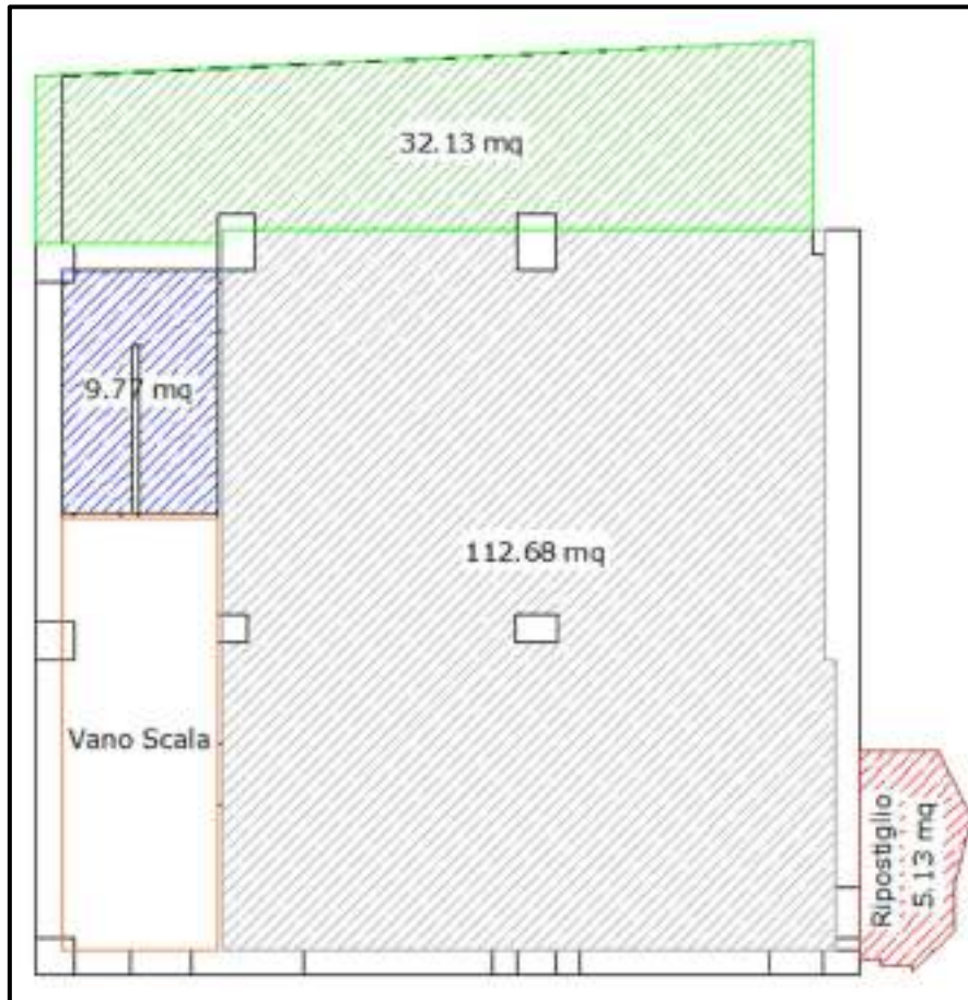
Fig. n. 13 – Stralcio planimetria del rilievo metrico eseguito in sede di sopralluogo
