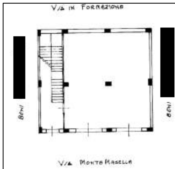
Fig. n. 12 – Stralcio visura e planimetria catastale
