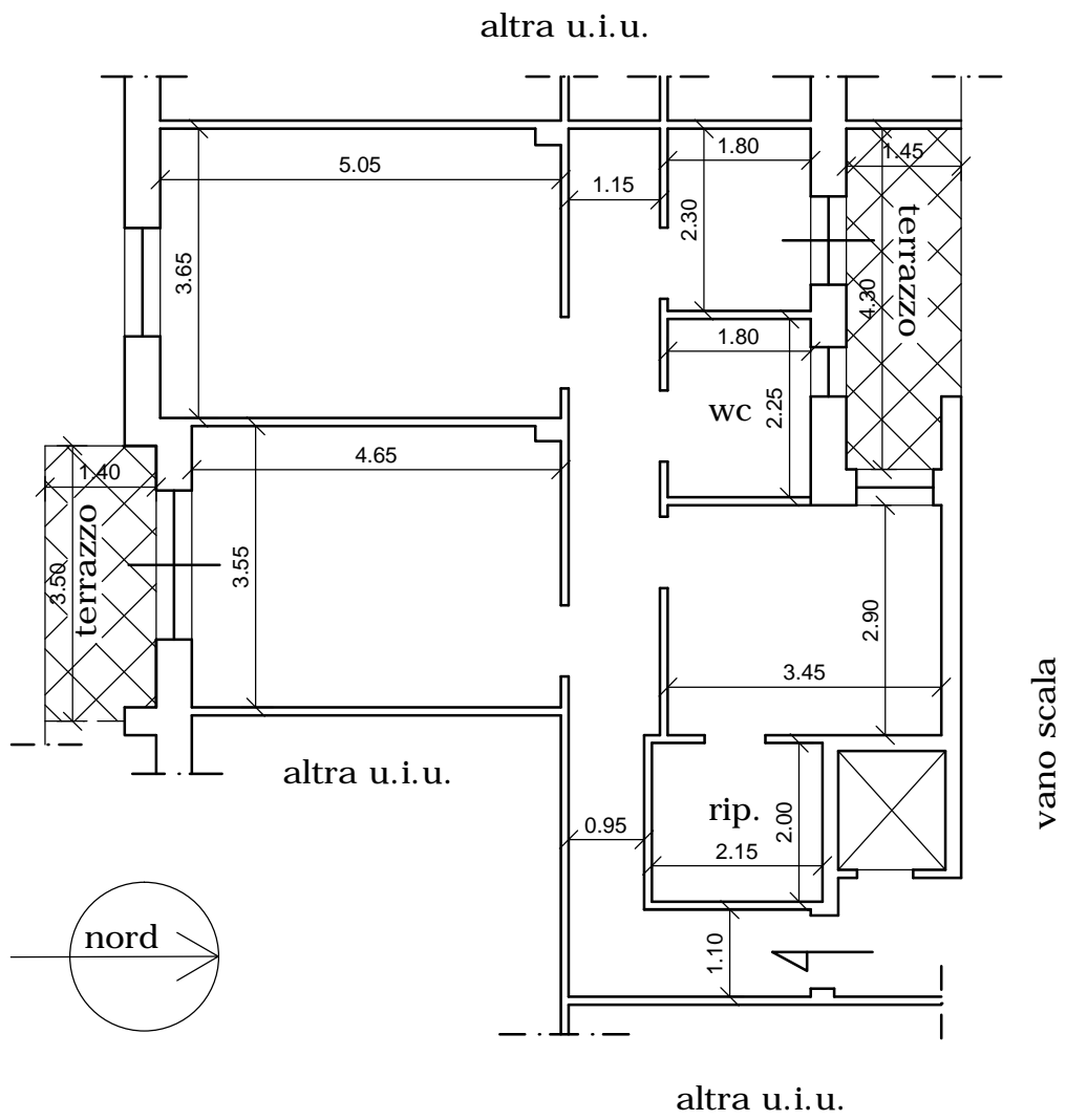
Pianta quotata appartamento stato attuale Piano 2° Scala B scala 1/100
