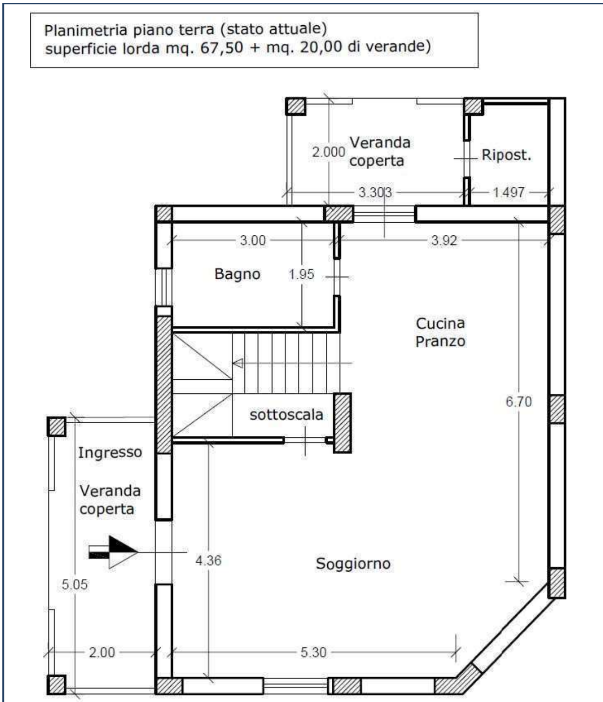
Planimetria stato ATTUALE piano Terra
