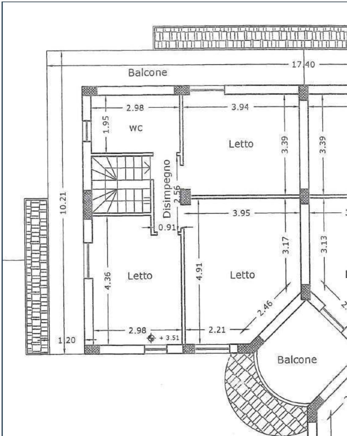
Planimetria progetto approvato – piano primo
