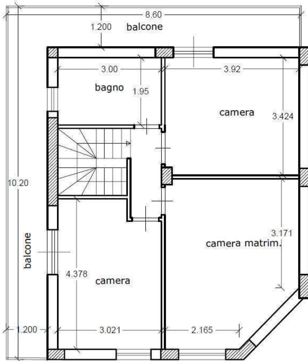
Planimetria stato ATTUALE piano Primo
