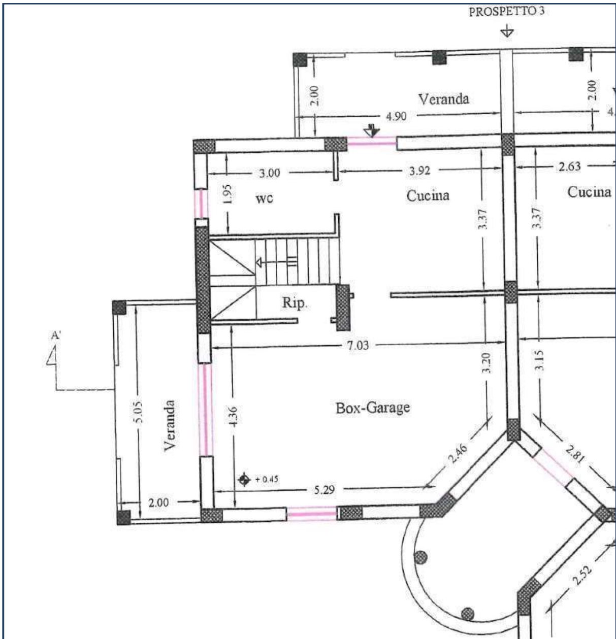
Planimetria progetto approvato – piano terra
