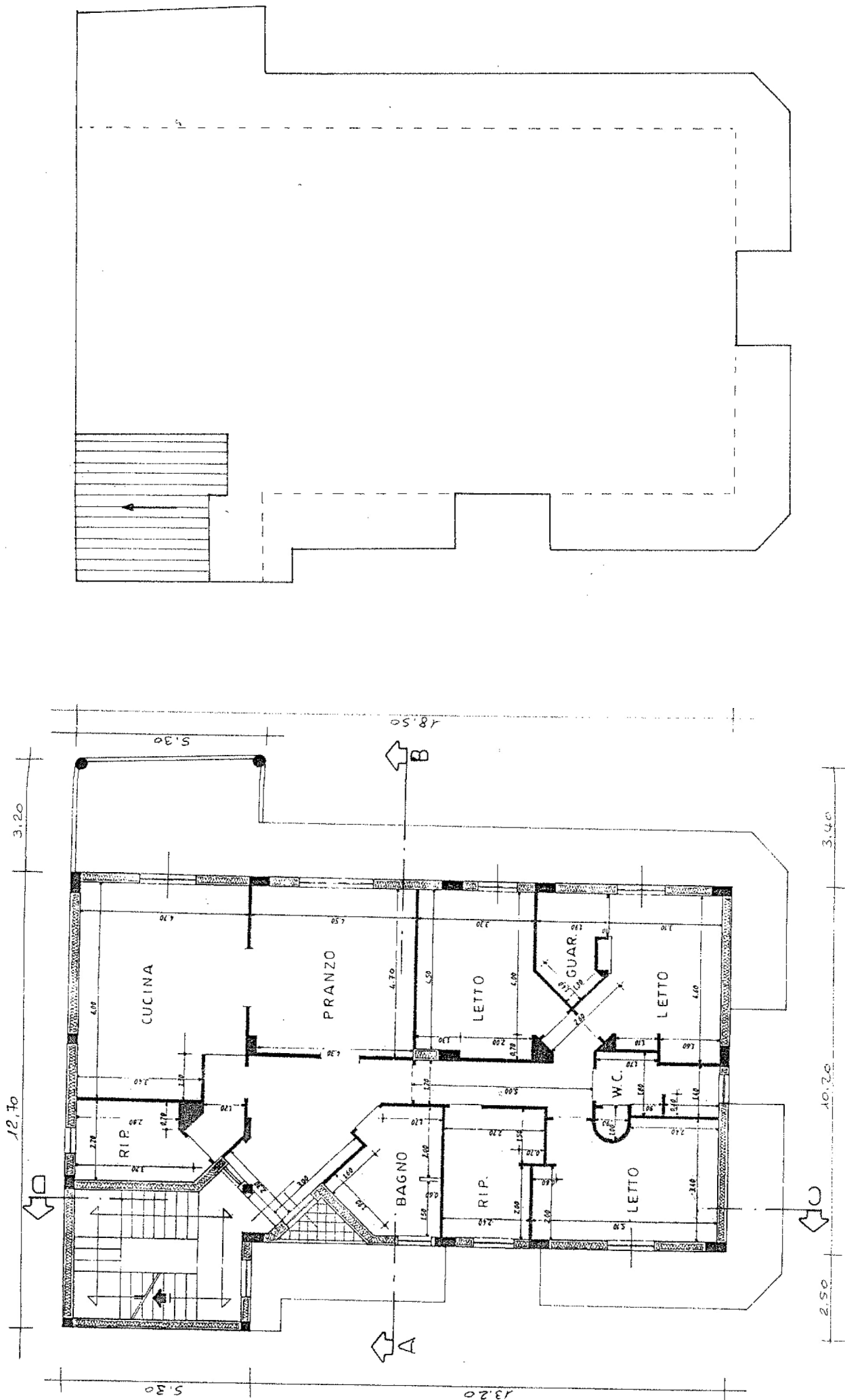
PIANTA PRIMO PIANO
