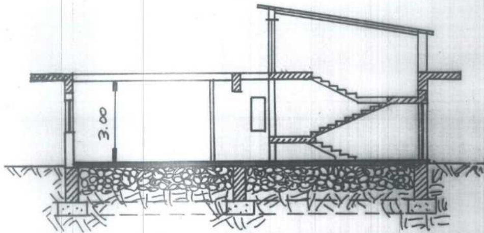
SEZIONE A:B scala 1:100
