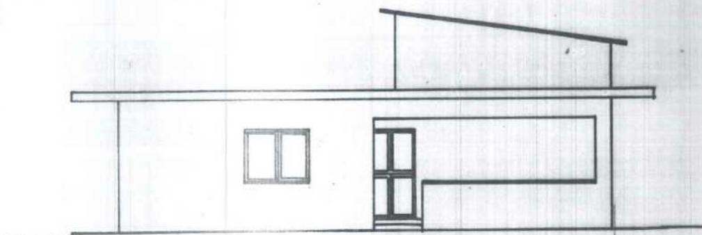
PROSPETTO LATO STRADA scala 1:100
