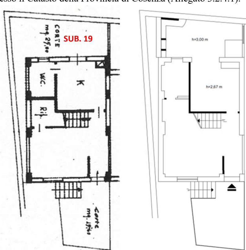
Immagine 3.2.5.1 – Confronto piano terra planimetria catastale depositata nel 1991 e stato di fatto
