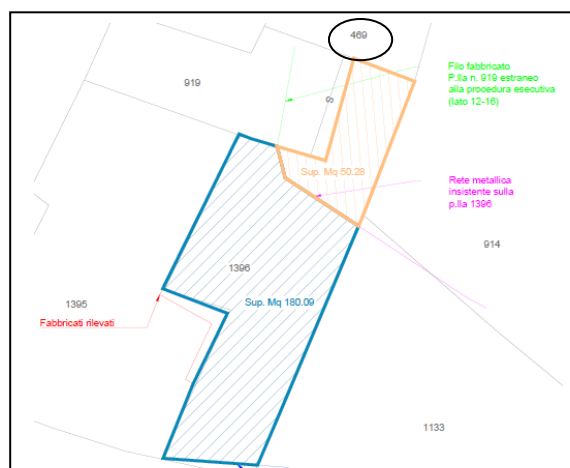
Restituzione grafica del rilievo eseguito con strumentazione gps
