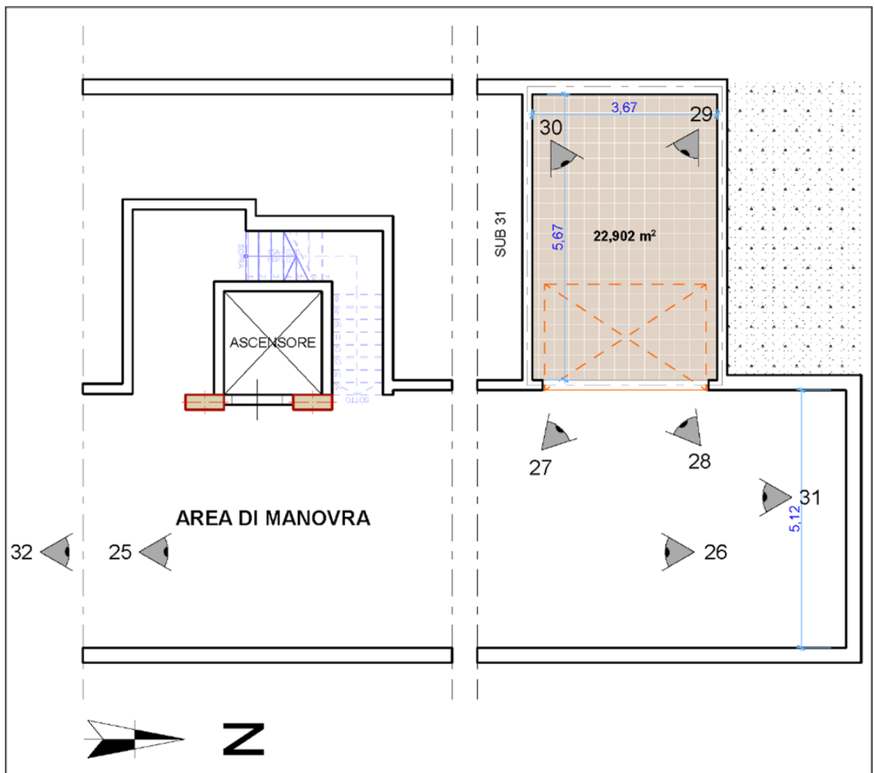
Planimetria stato di fatto box - con ottici
