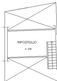
PIANTA PIANO QUINTO
