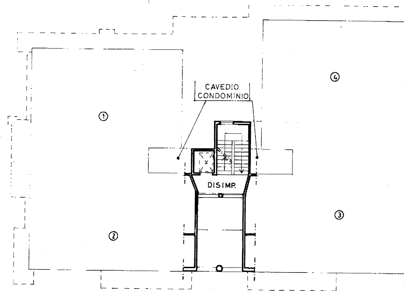
PIANO PRIMO SCALA 1:200 H = 2.70
