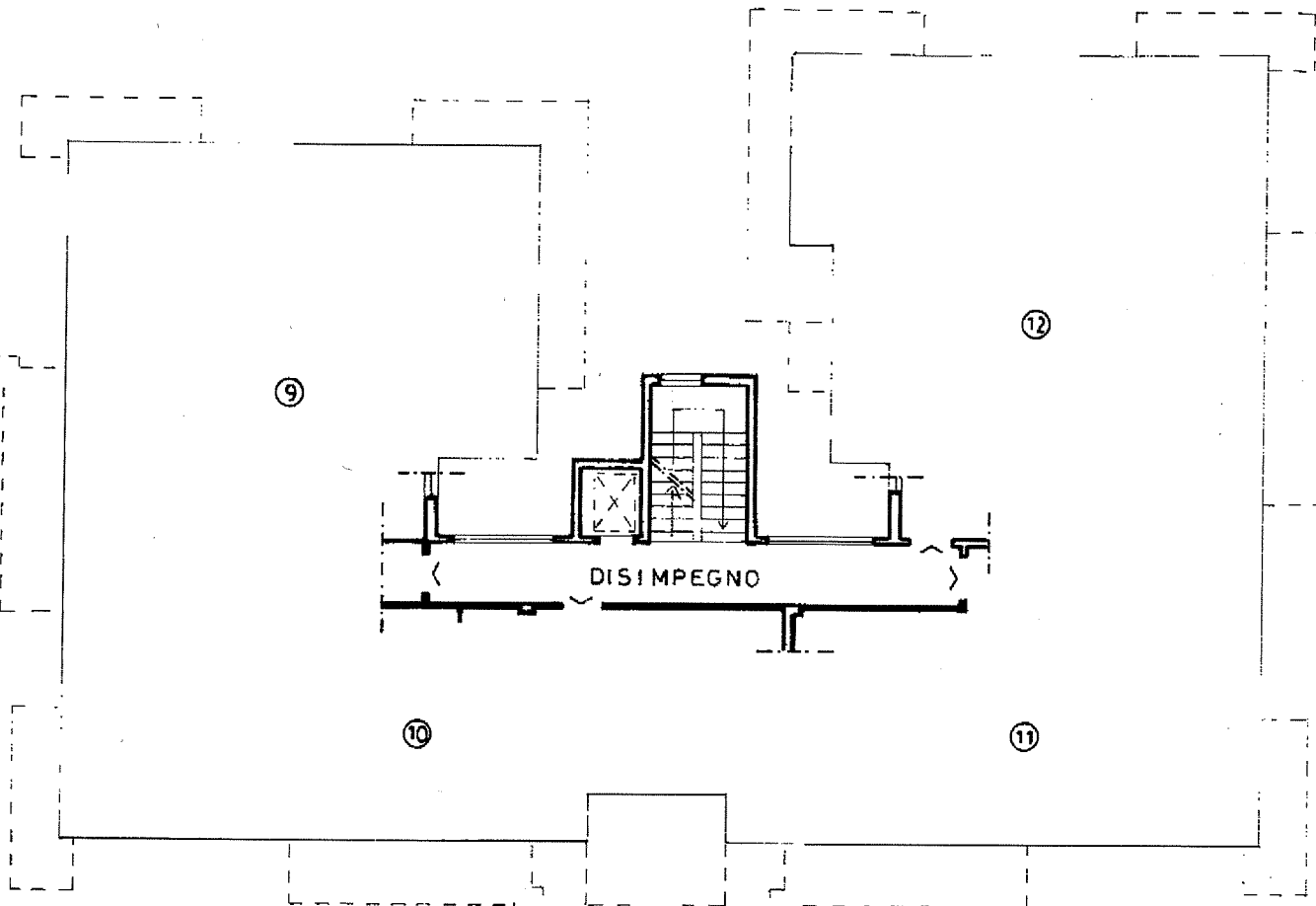
PIANO TERZO SC. 1 200 H= 2.70
