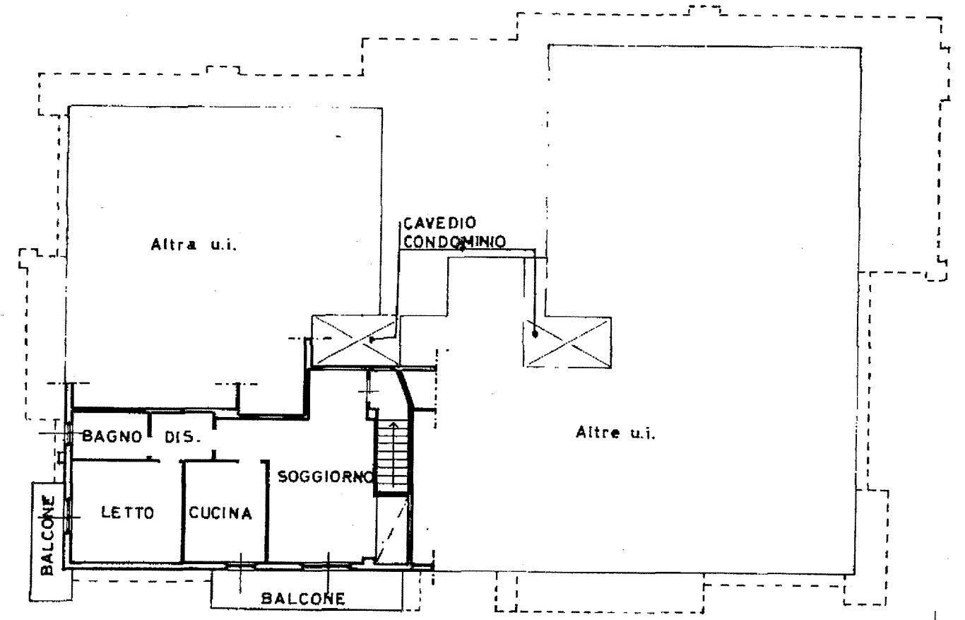
PIANO PRIMO H = 2.70
