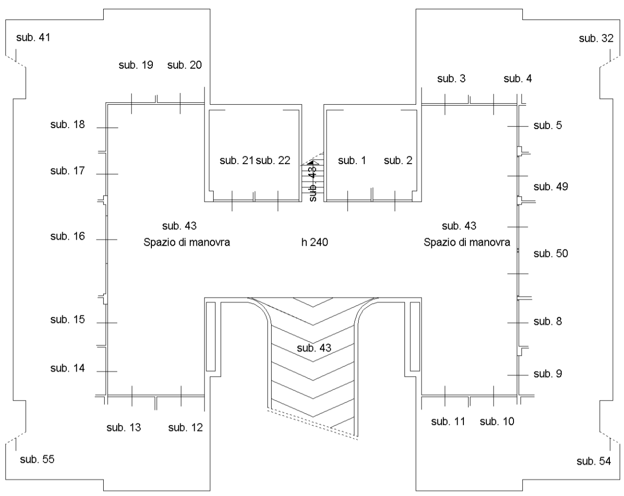
Piano Primo Sottostrada h 240
