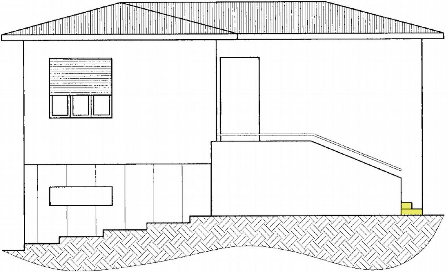
PROSPETTO SU VIA SANTERNO AMMONITE
