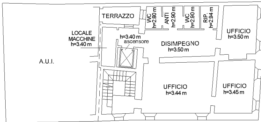
PIANO PRIMO
