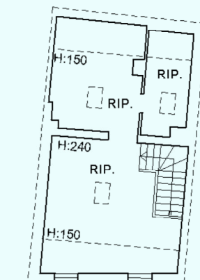
PIANO SECONDO -sottotetto
