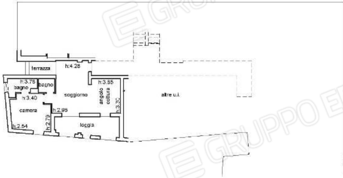
Fabbricato B Piano Terzo
