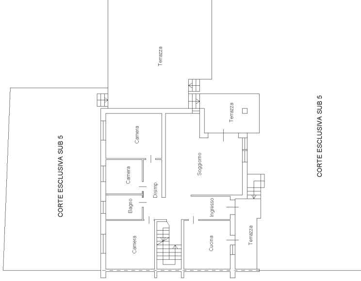
PIANTA PIANO TERRA H = 3,20
