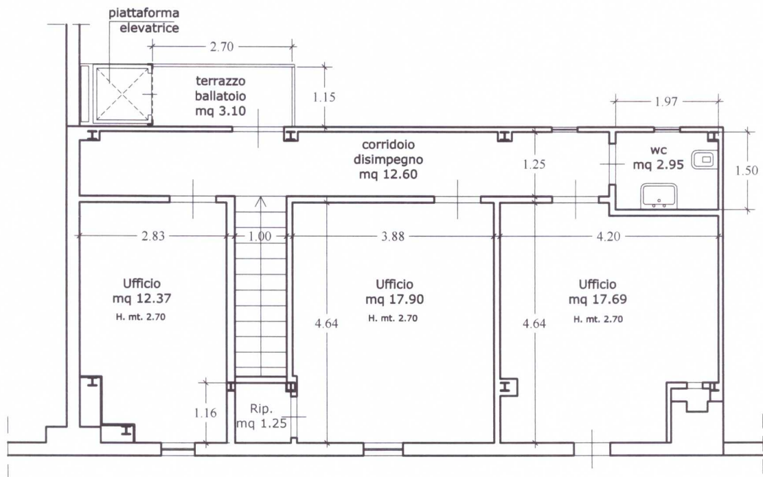
PLANIMETRIA - PIANO PRIMO RILIEVO STATO ATTUALE RAPP. 1:100
