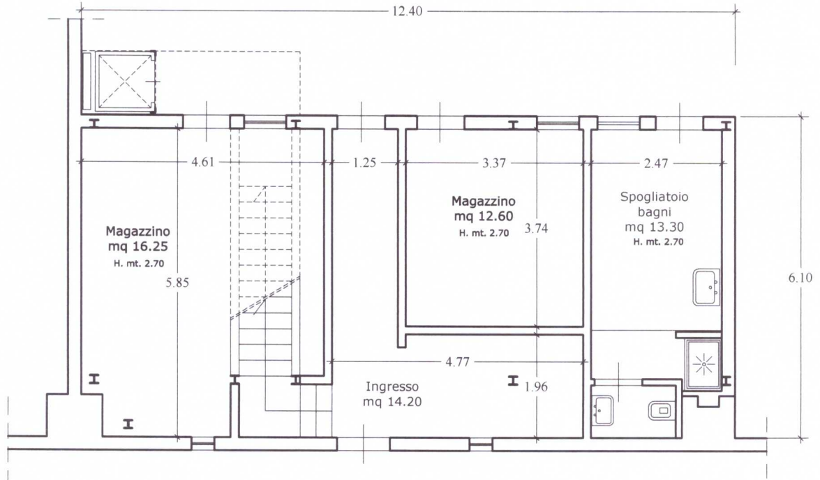
PLANIMETRIA - PIANO TERRA RILIEVO STATO ATTUALE RAPP. 1:100
