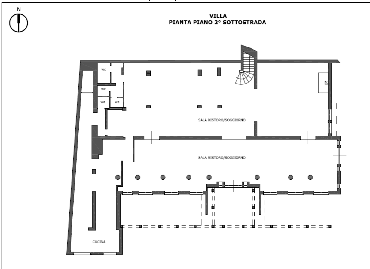
Rilievo pianta piano 2° sottostrada
