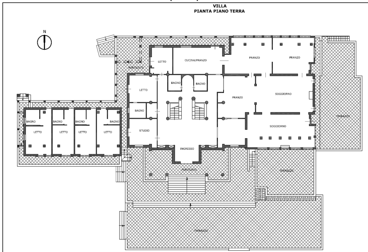
Rilievo pianta piano terra
