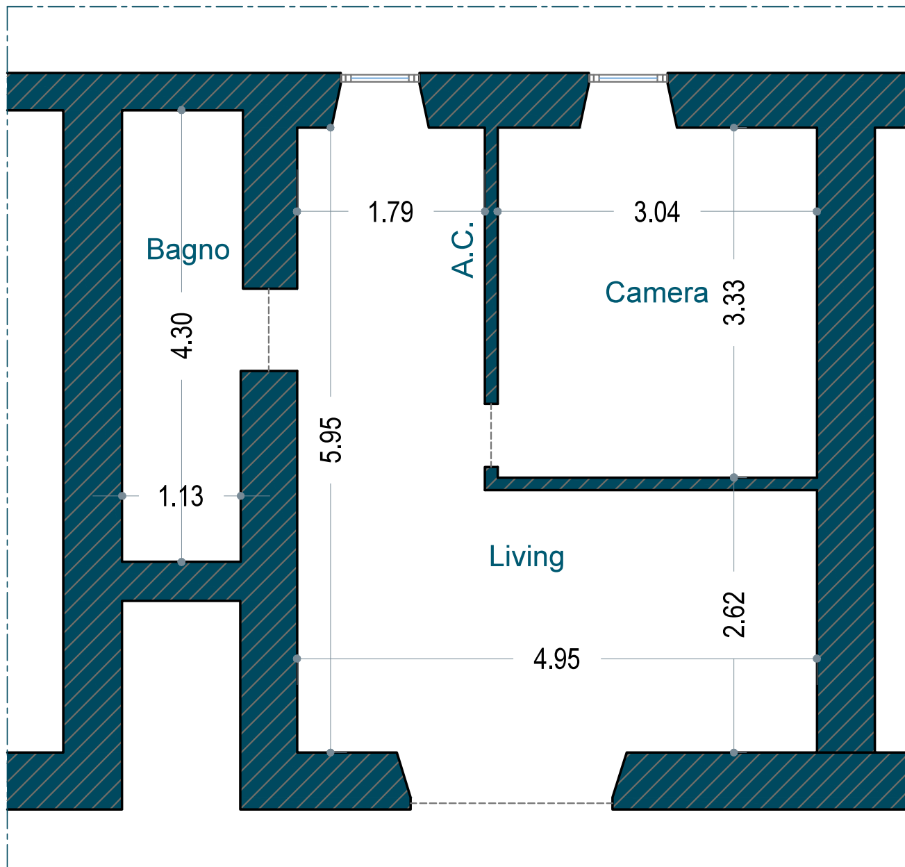
PIANTA REALE PIANO TERRA
