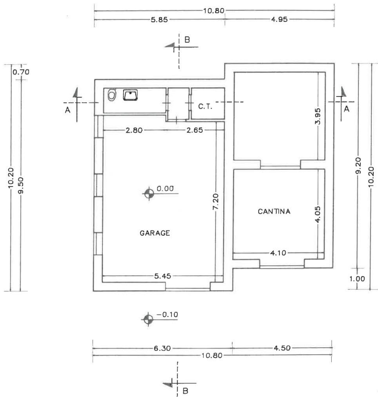
PIANTA PIANO SEMINTERRATO
