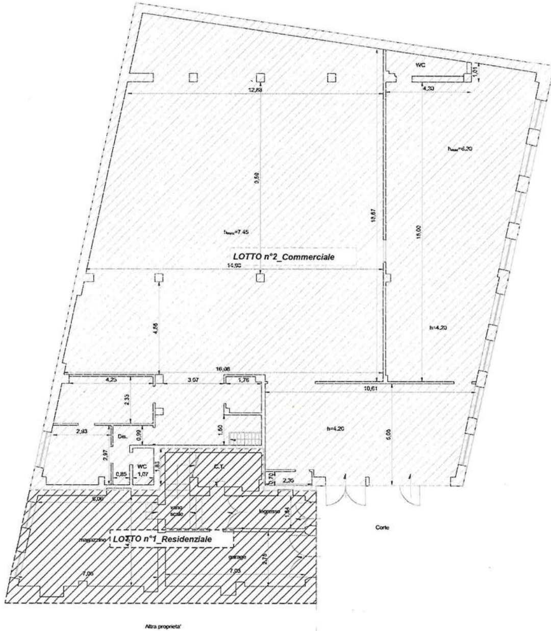
Pianta Piano Terra - Scala 1:100
