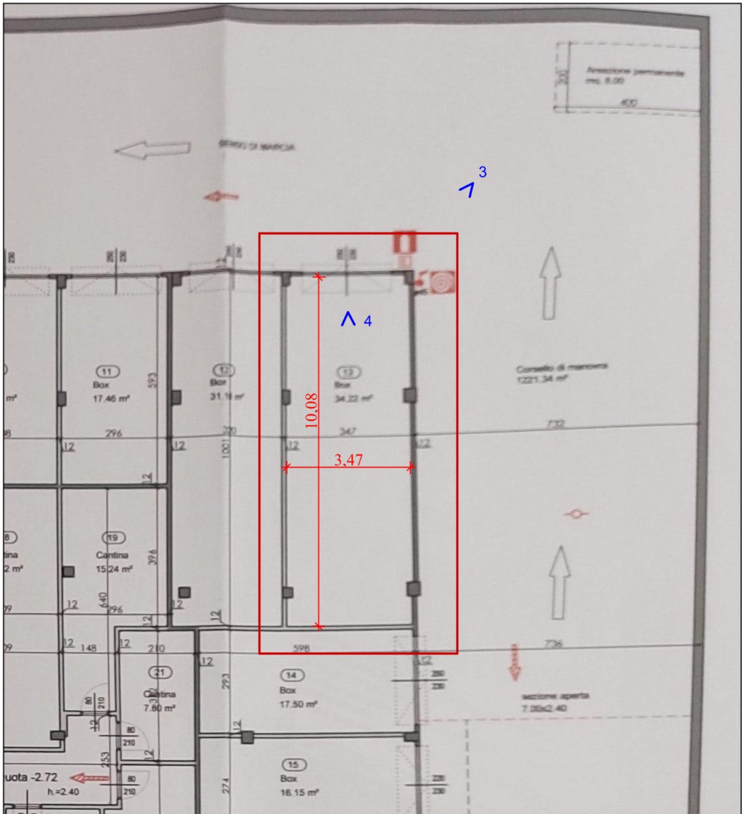
PIANTA PIANO INTERRATO Permesso di Costruire numero 11 del 11/10/2007 e successive varianti
