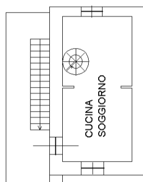
PIANO SECONDO H 260
