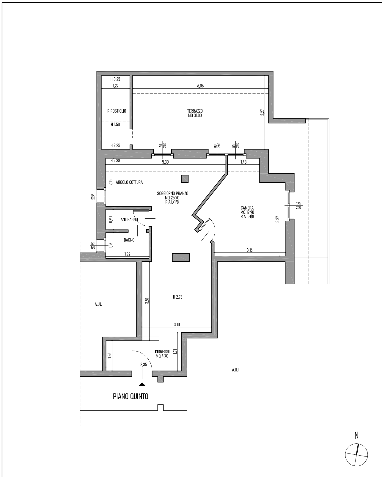
Appartamento in via Europa n. 3 - LEFFE (BG) PIANTA PIANO QUINTO - SCALA 1:100
