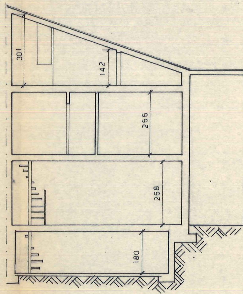
sezione aa
