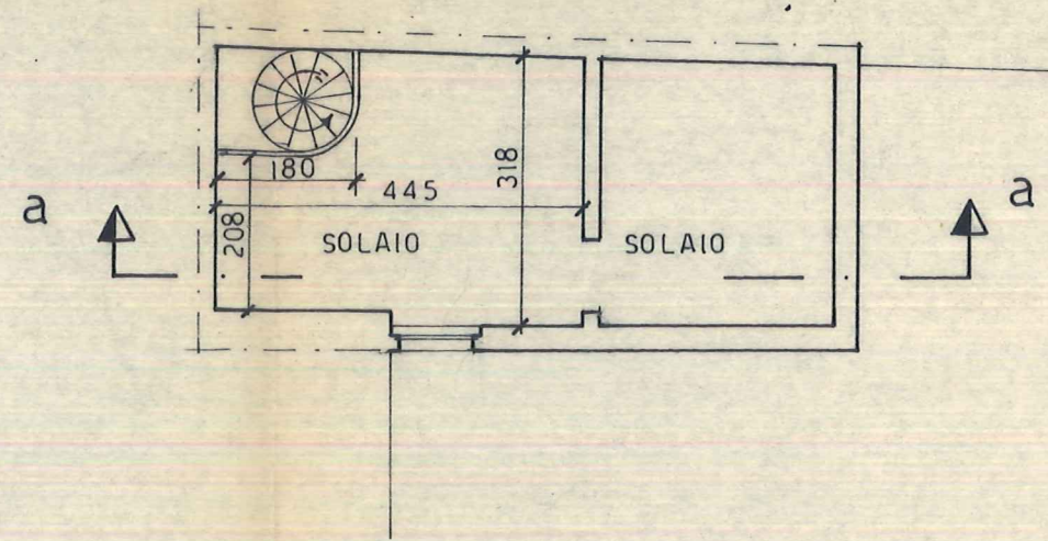
piano sottotetto
