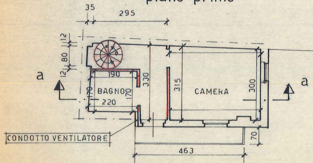
piano primo
