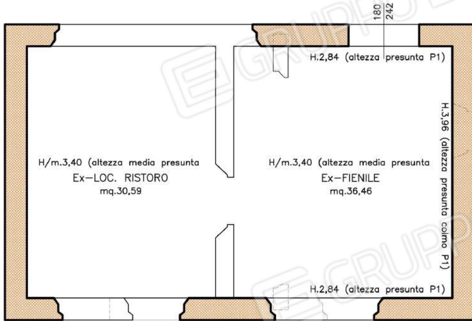
PIANO PRIMO
