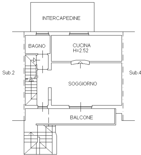
PIANO RIALZATO (T.) H.= 275
