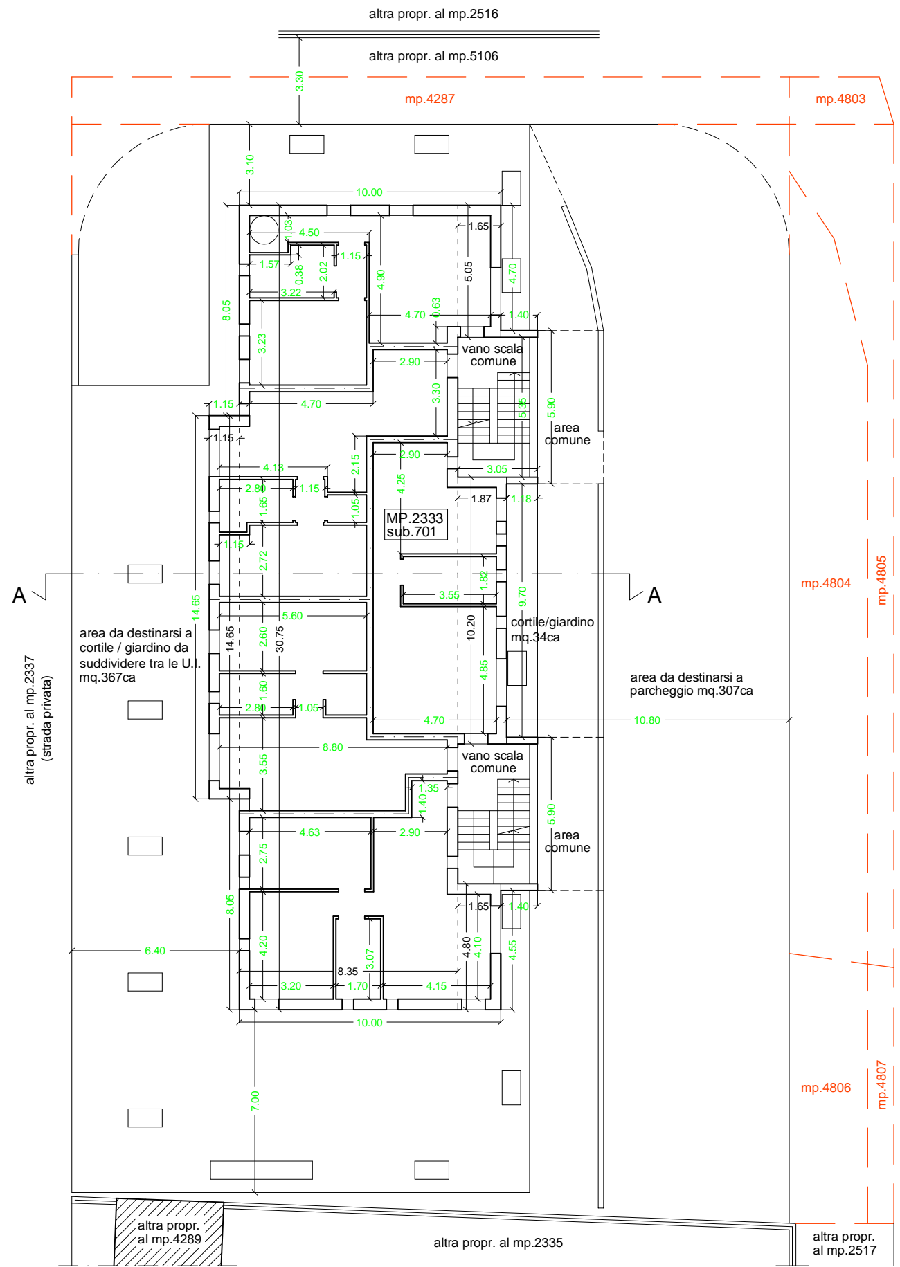
PIANTA p.TERRA
