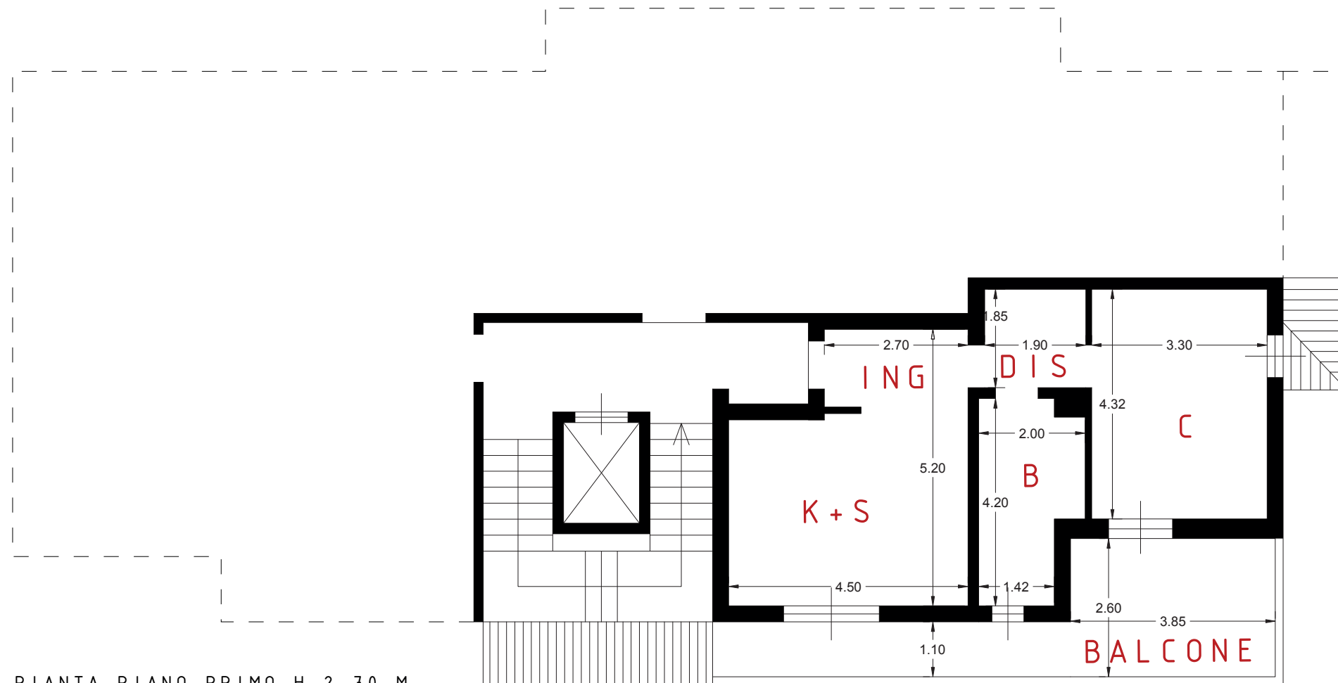
PIANTA PIANO PRIMO H 2.70 M
