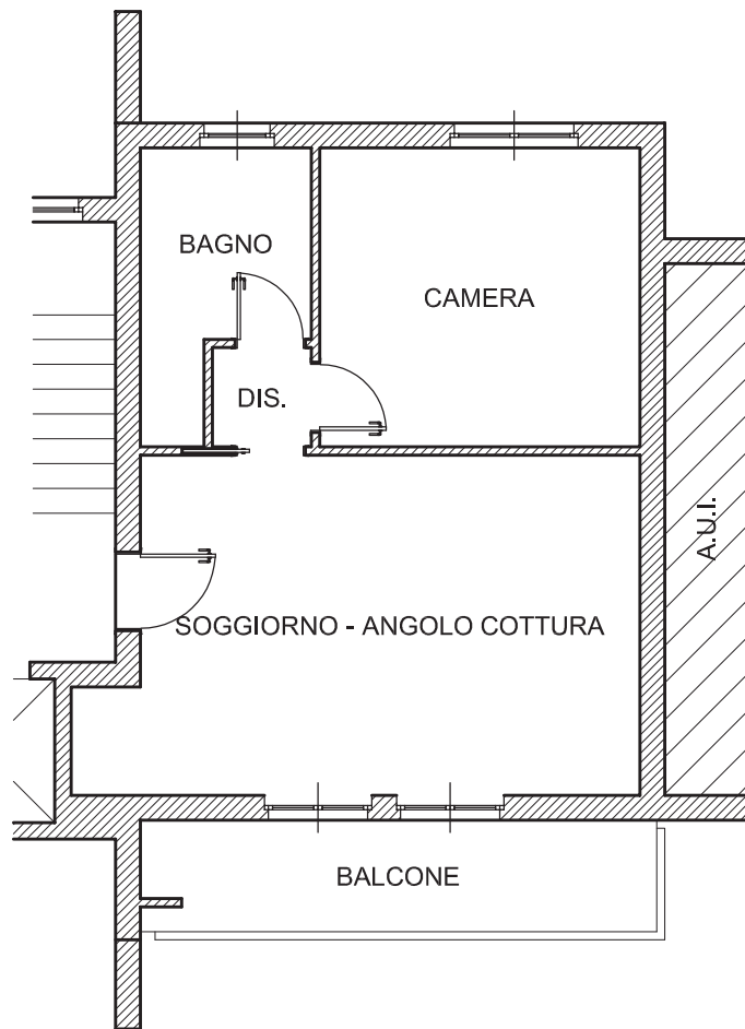
PIANTA PIANO PRIMO H=2.70 m
