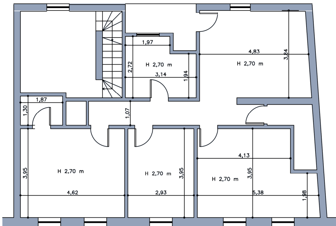
PIANO PRIMO
