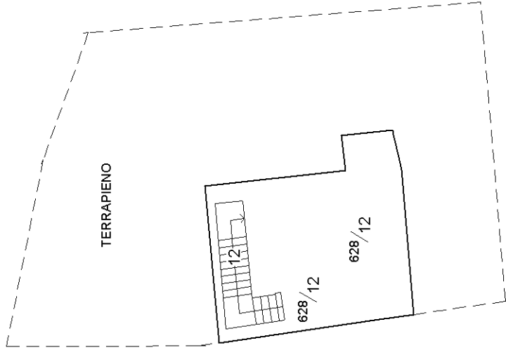
PIANO PRIMO SOTTOSTRADA (S1)
