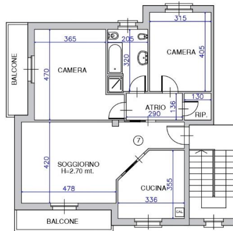
PIANO PRIMO sub.7
