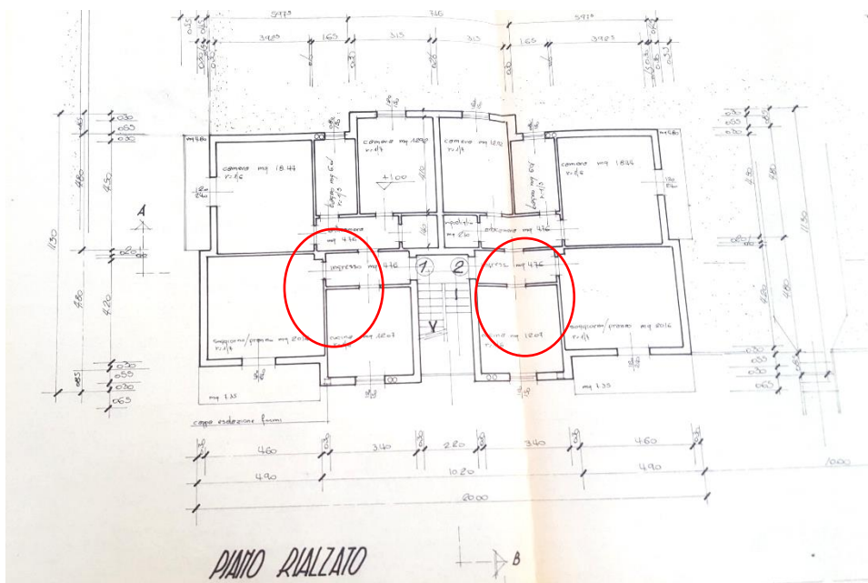
VIA SAN ROCCO Schema delle difformità a piano terra
