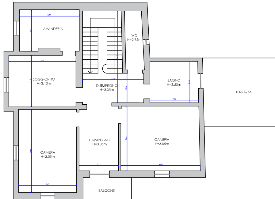
PIANTA PIANO PRIMO Foglio 194, mapp.14
