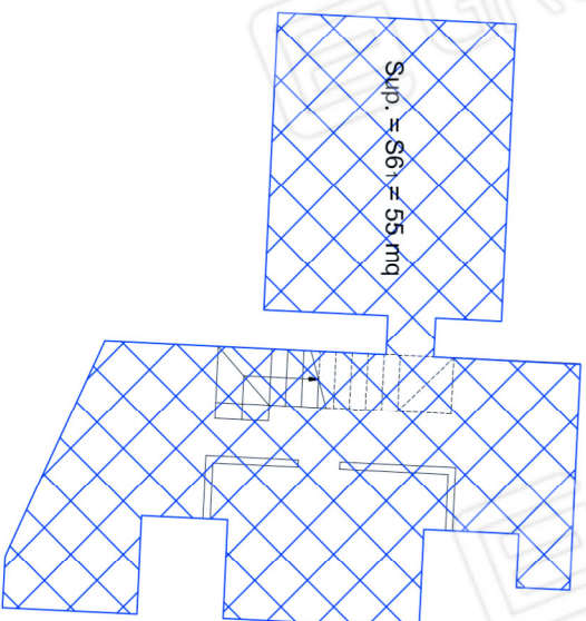
PIANTA PIANO INTERRATO (cantina) sc. 1:100
