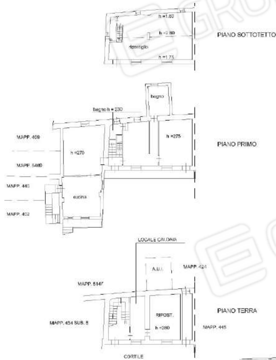
Planimetrie abitazione
