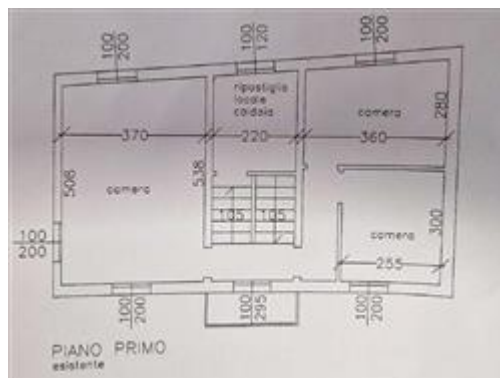
stato tavola di progetto pratica del 2002 dopo la sanatoria privo della scala di accesso al piano secondo sottotetto
