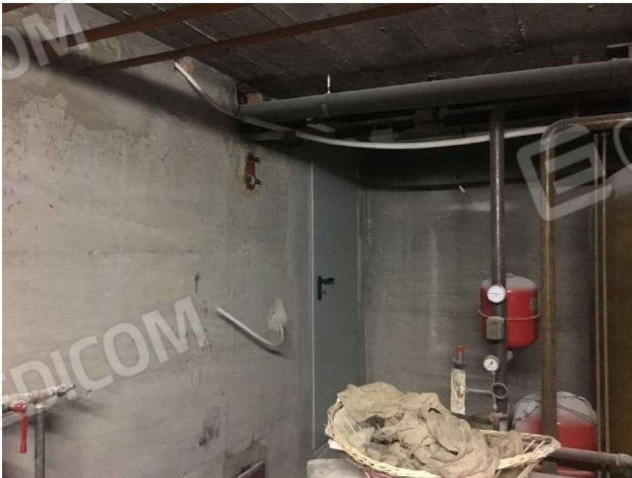
21. DETTAGLIO OPERE SVOLTE: nuovo accesso REI al locale caldaia
