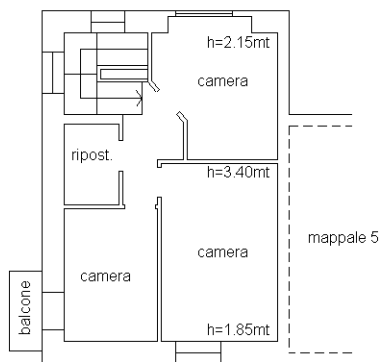
PIANO SECONDO h med.=2.65mt
