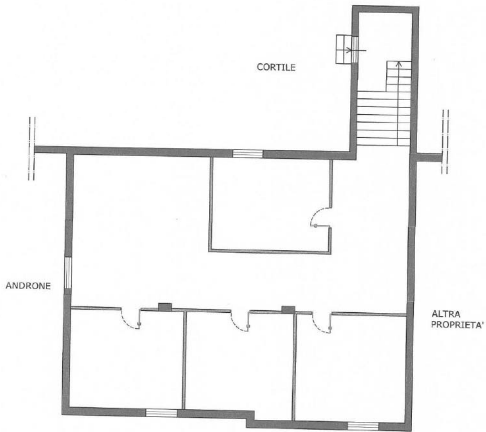
PIANTA PIANO SEMINTERRATO sub.9 scala 1:100
