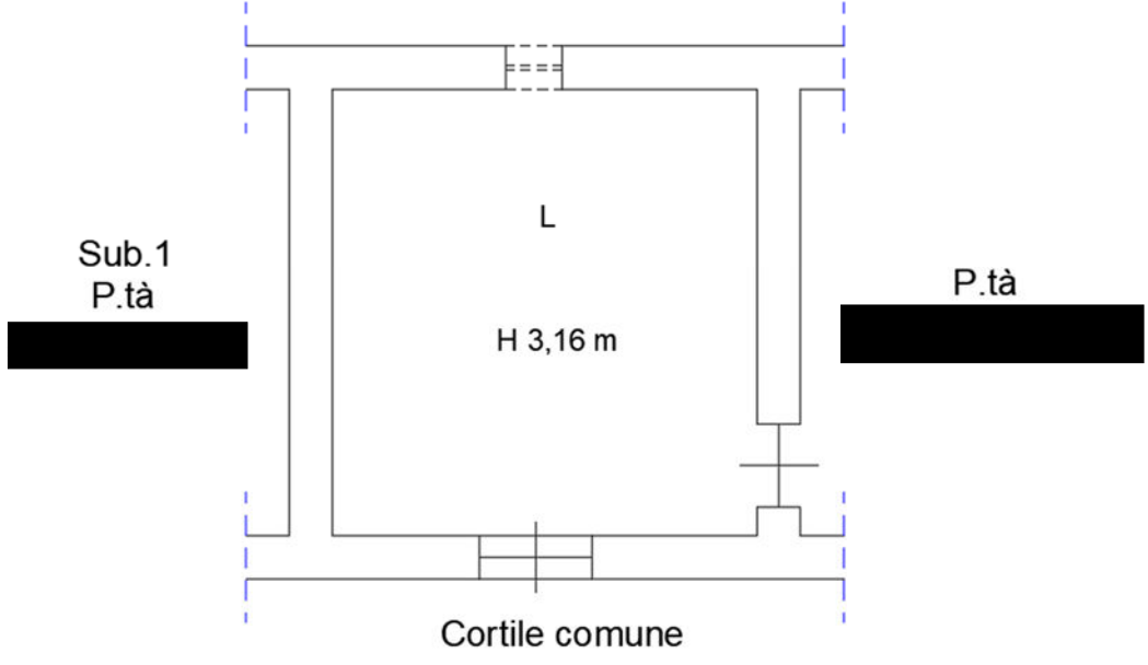
Planimetria piano terra sub.8 stato reale
