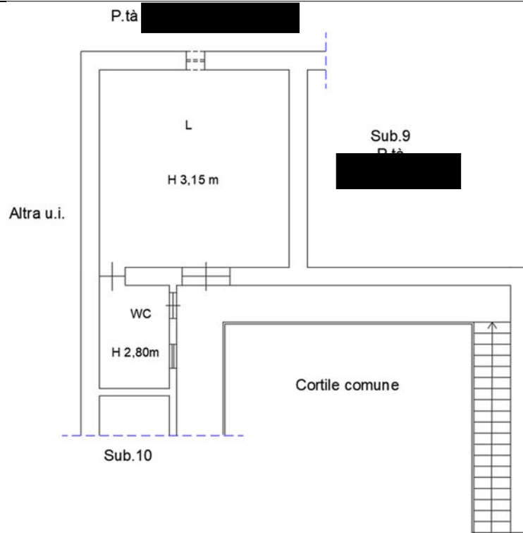
Planimetria piano primo sub.5 stato reale
